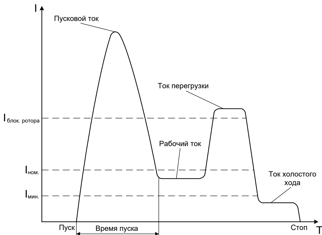
Рисунок В.1 - Диаграмма соотношений уровней запрограммированных и протекающих в электродвигателе токов
